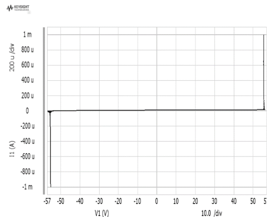
Figure4: I-V Curve
